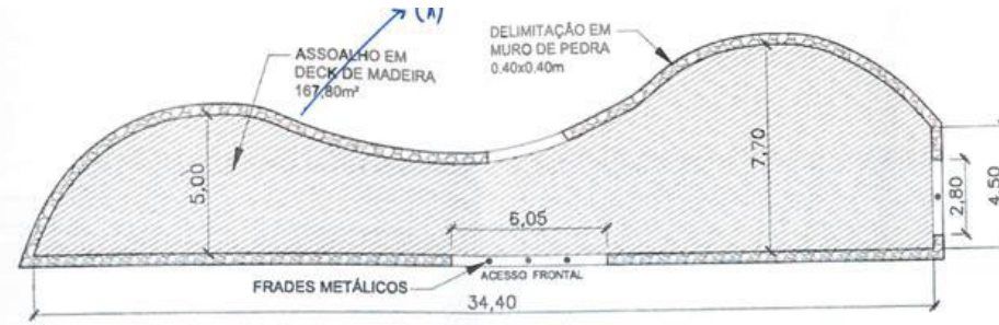
2 PLANTA BAIXA ESQUEMÁTICA – DECK ILHA 05 ESC. 1:200
