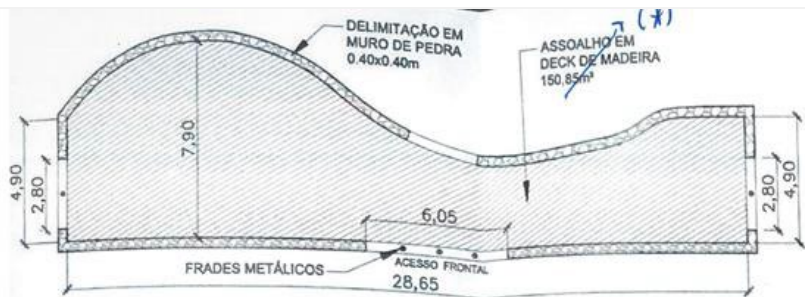
1 PLANTA BAIXA – DECKS ILHA 26/24/19/17 E 08 ESC. 1:200
