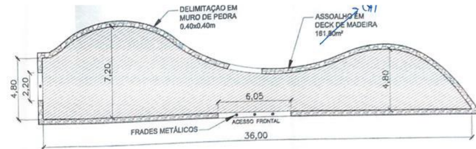
4 PLANTA BAIXA ESQUEMÁTICA – DECK ILHA 04 ESC. 1:200
