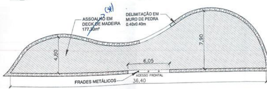
1 PLANTA BAIXA – DECKS ILHA 26/24/19/17 E 08 ESC. 1:200
